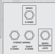
GB 412G-FLEX パネル
