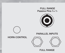
XB2 シリーズ リアパネル
