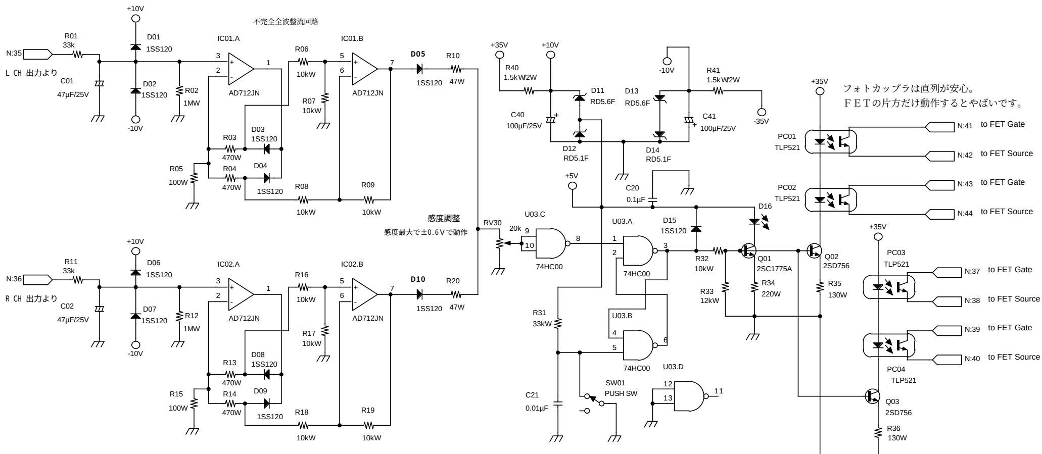
金田式UHC POWER AMP用保護回路
