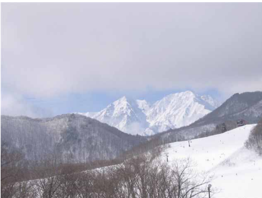
杓子岳と白馬鑓ヶ岳
