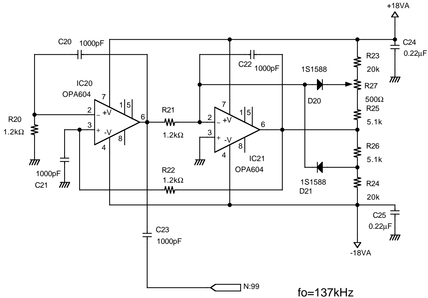
バイアス発振器に用いたクワドラチャ発振器
