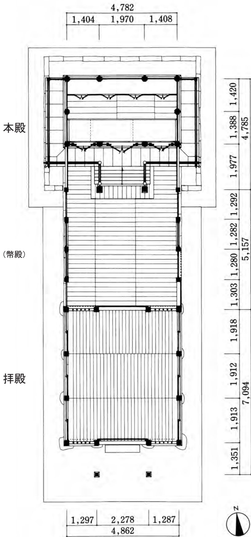
本殿・拝殿平面図
