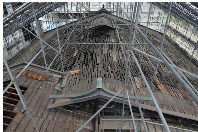
板葺きは撤去し、野地の補修等を行った後、葺替えを行う予定です。
