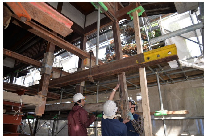
柱で蟻害が著しく再用が困難な一部のものは取替を行いました。
