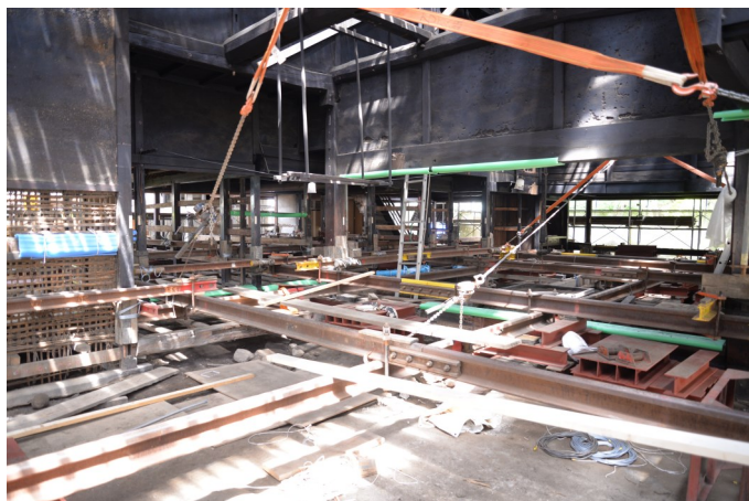
揚屋を行うため各所にレール材を設置して柱を固めました。
