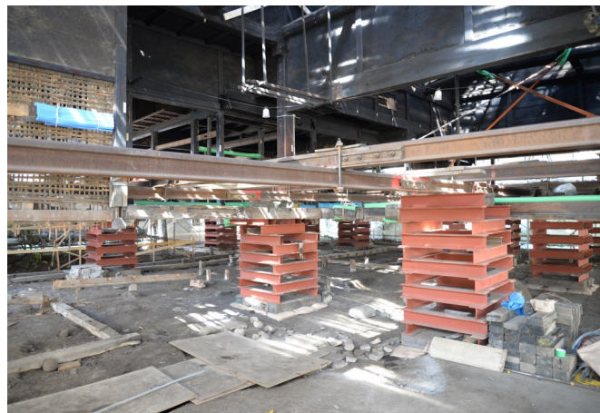
建物を地上から1.3m揚げて土台・柱の補修を行いました。
